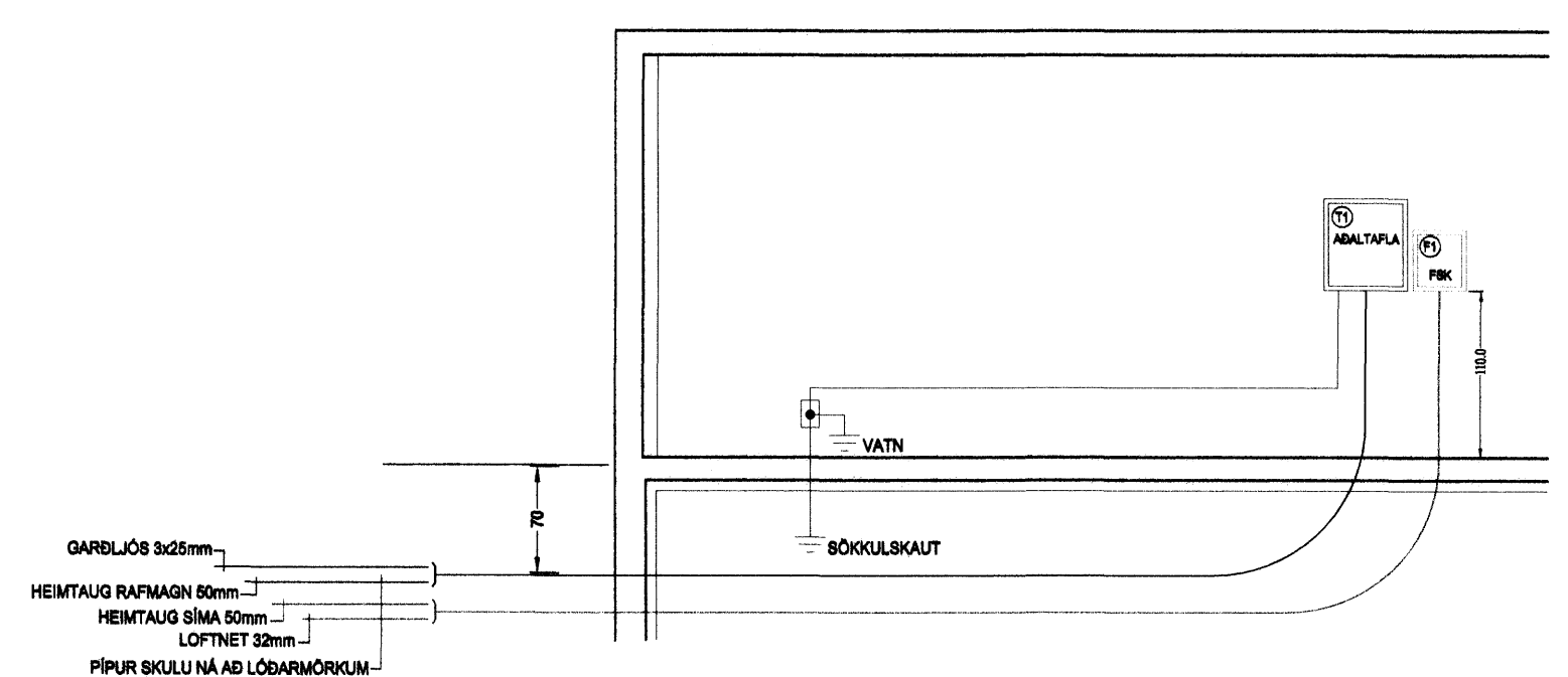
SNIÐ A-A MKV. 1:50
