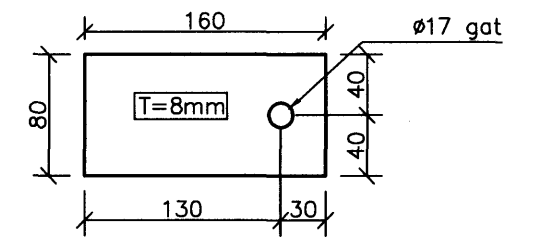
EYRA-A 1:5
