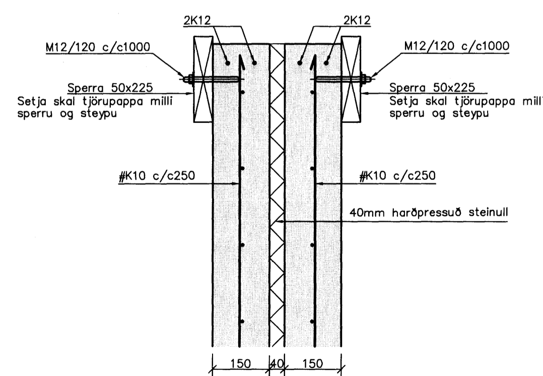
DEILI 1:10 C B06
