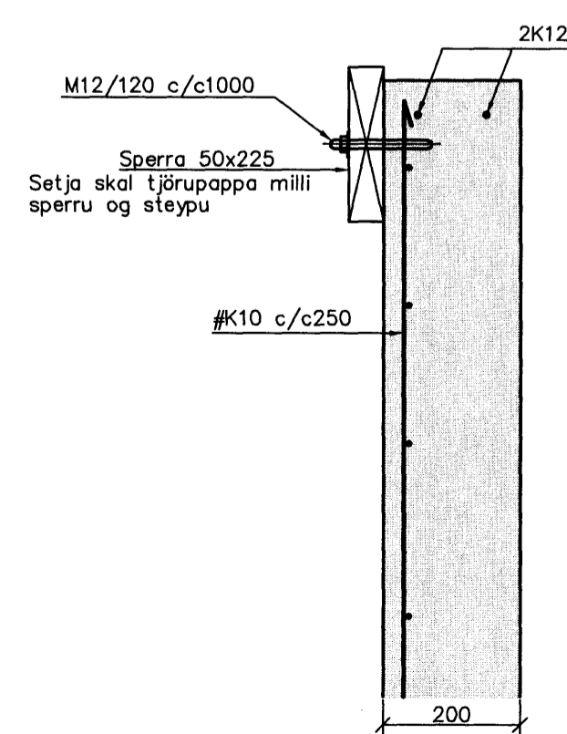
DEILI 1:10 B B06
