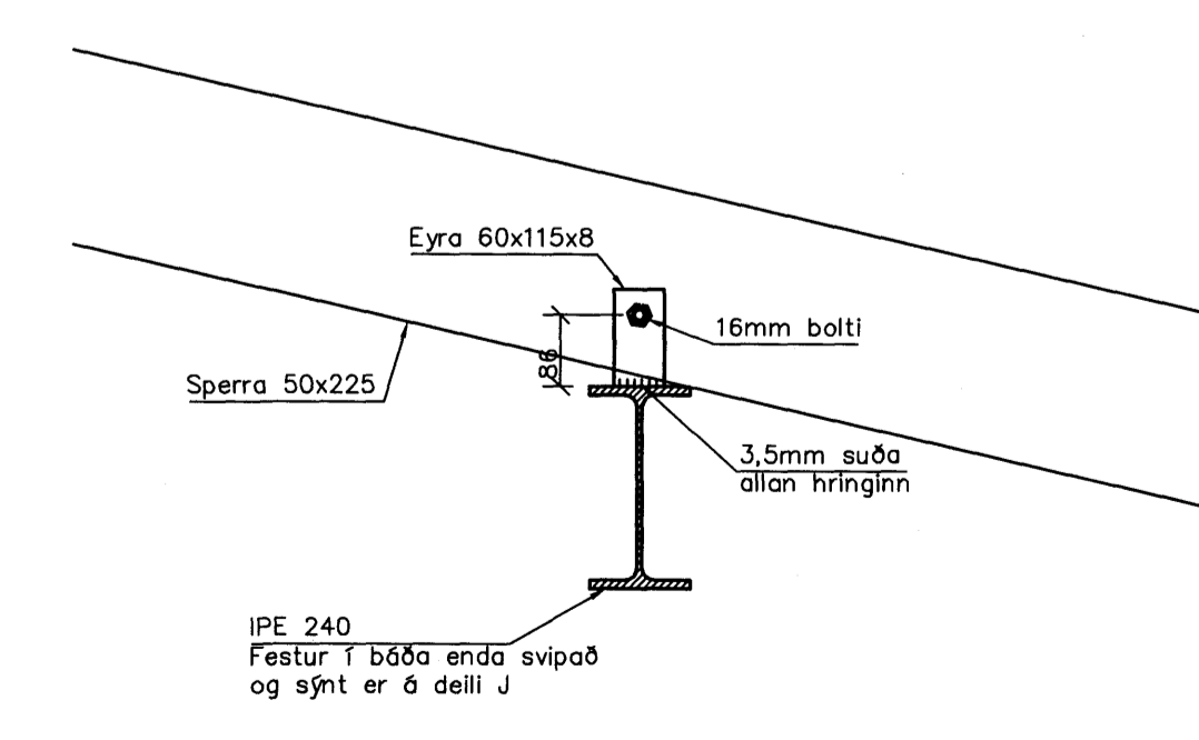
DEILI 1:10 E B06
