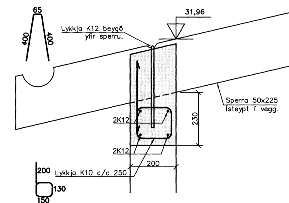
DEILI 1:10 D B06
