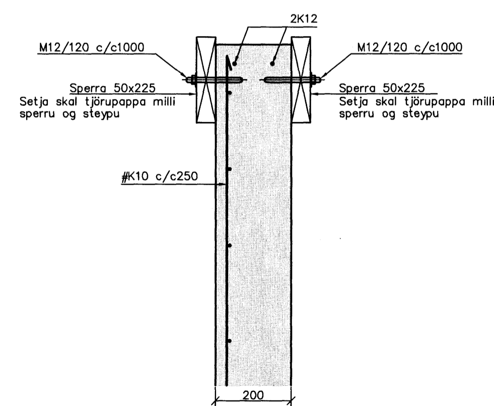
DEILI 1:10 A B06
