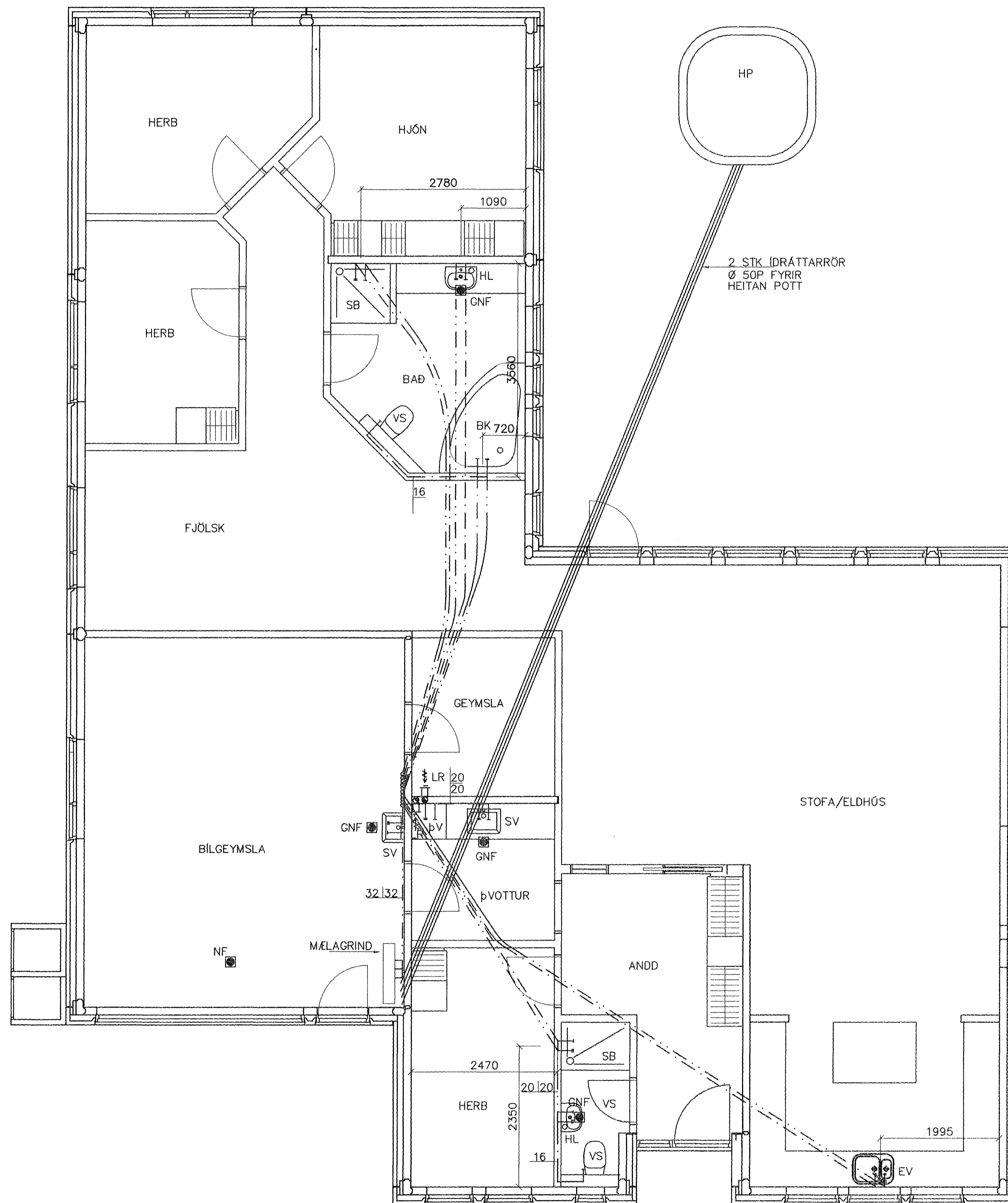
GRUNNMYND 1:50
