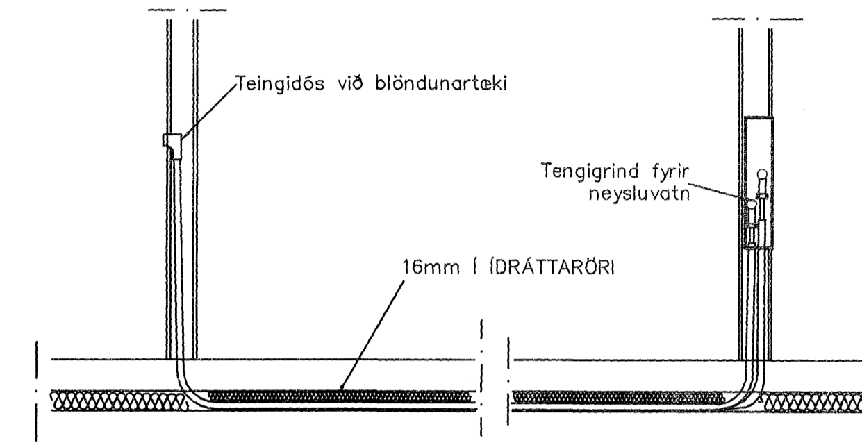
TENING NEYSLUVATNSLAGNA 1:20
