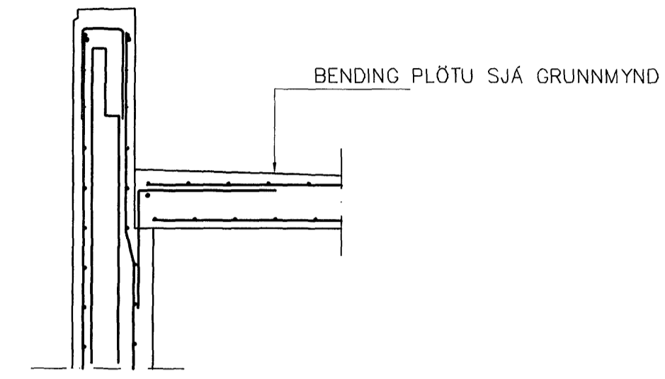
SNID 1-1 1:20
