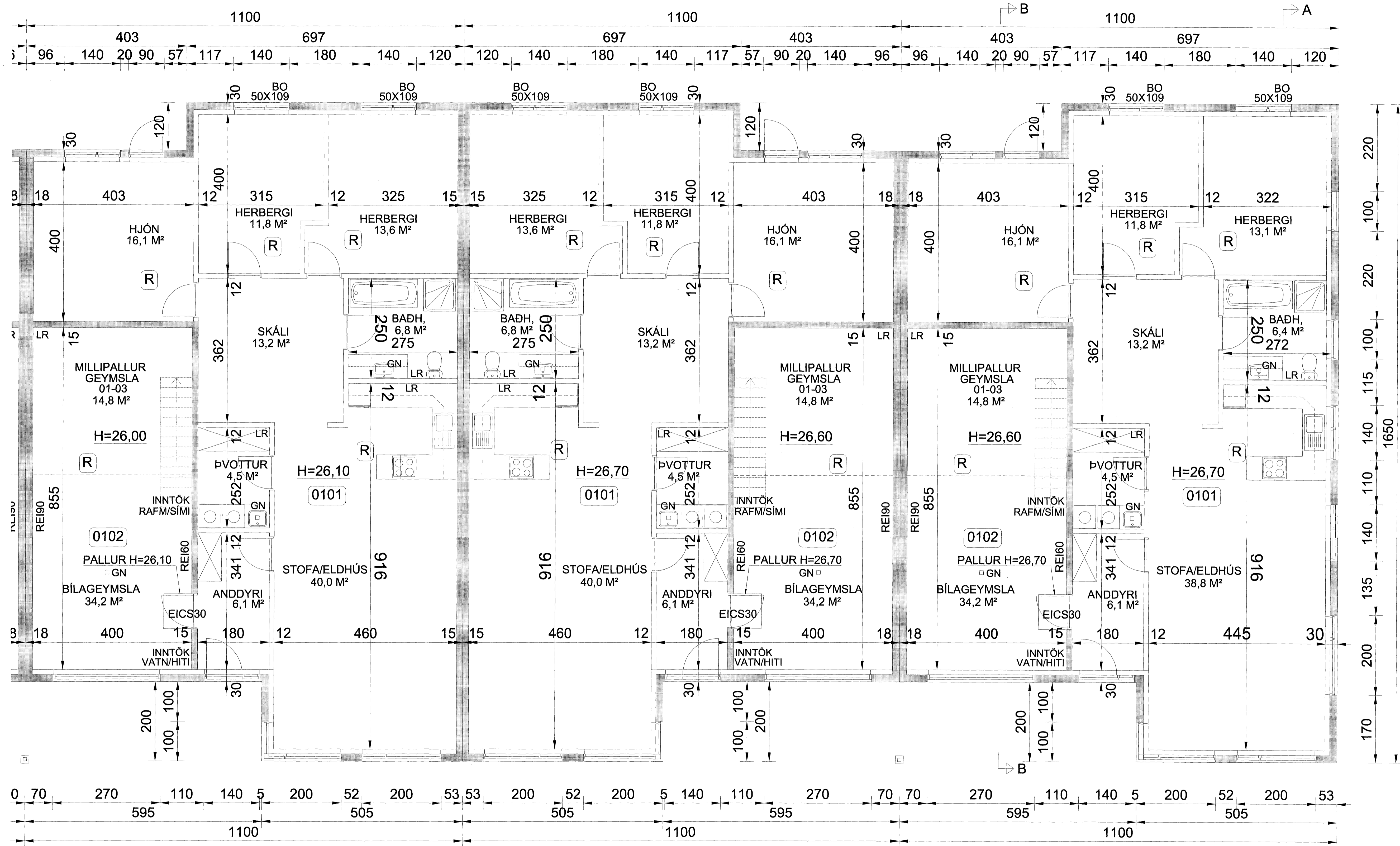
HÚS NR. 27, 29 OG 31 GRUNNMYND 1:50
