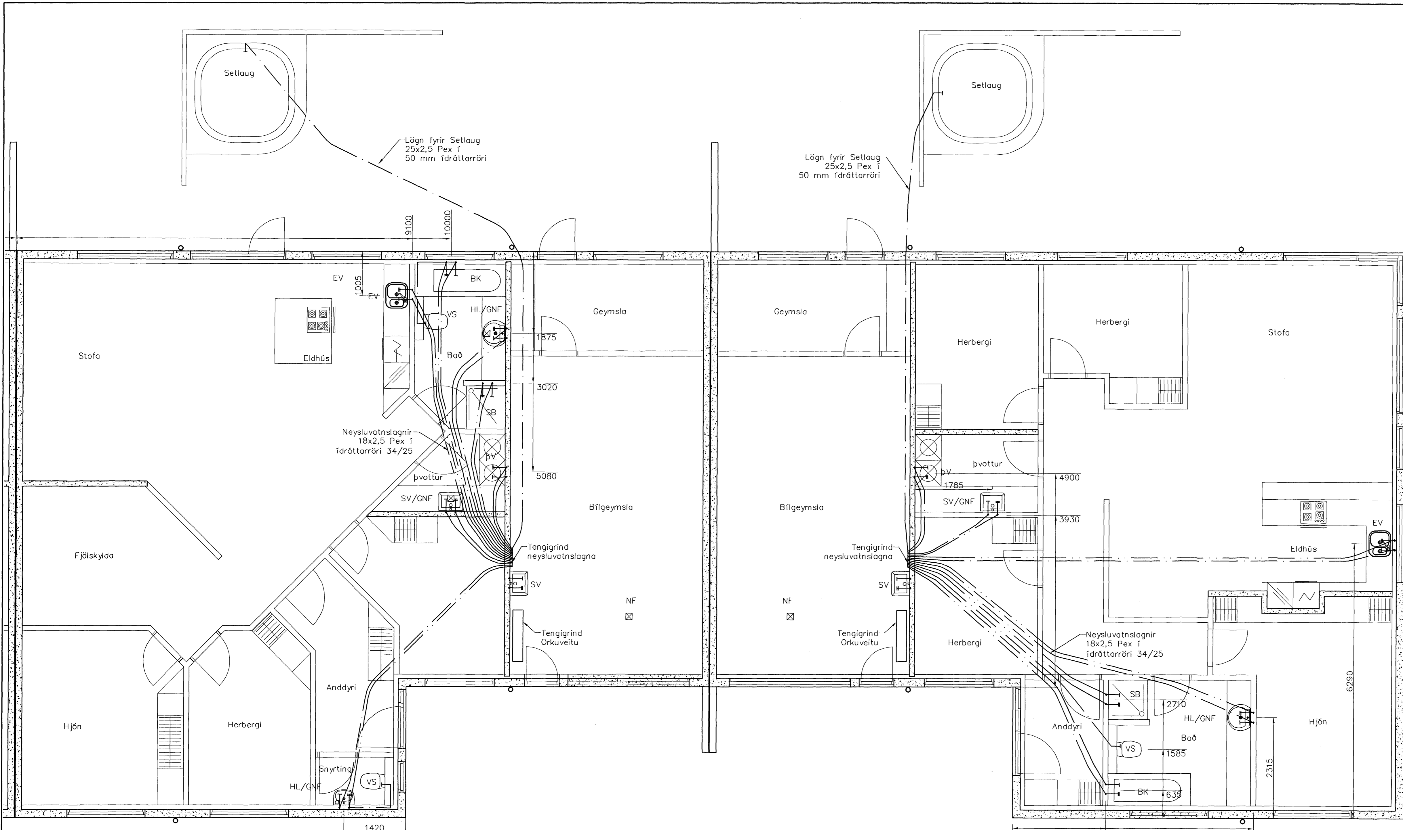
Neysluvatnslagnir 1:50
