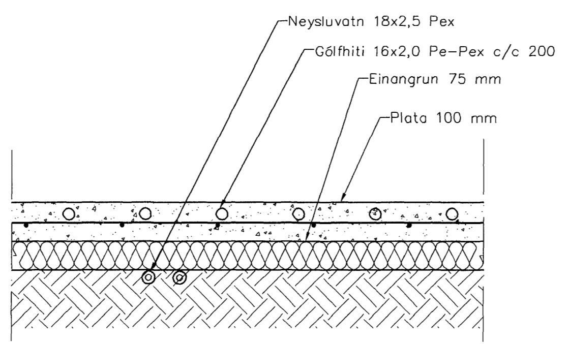
Hita- og vatnslagnir. Snið í botnplötu, íbúð 1:10
