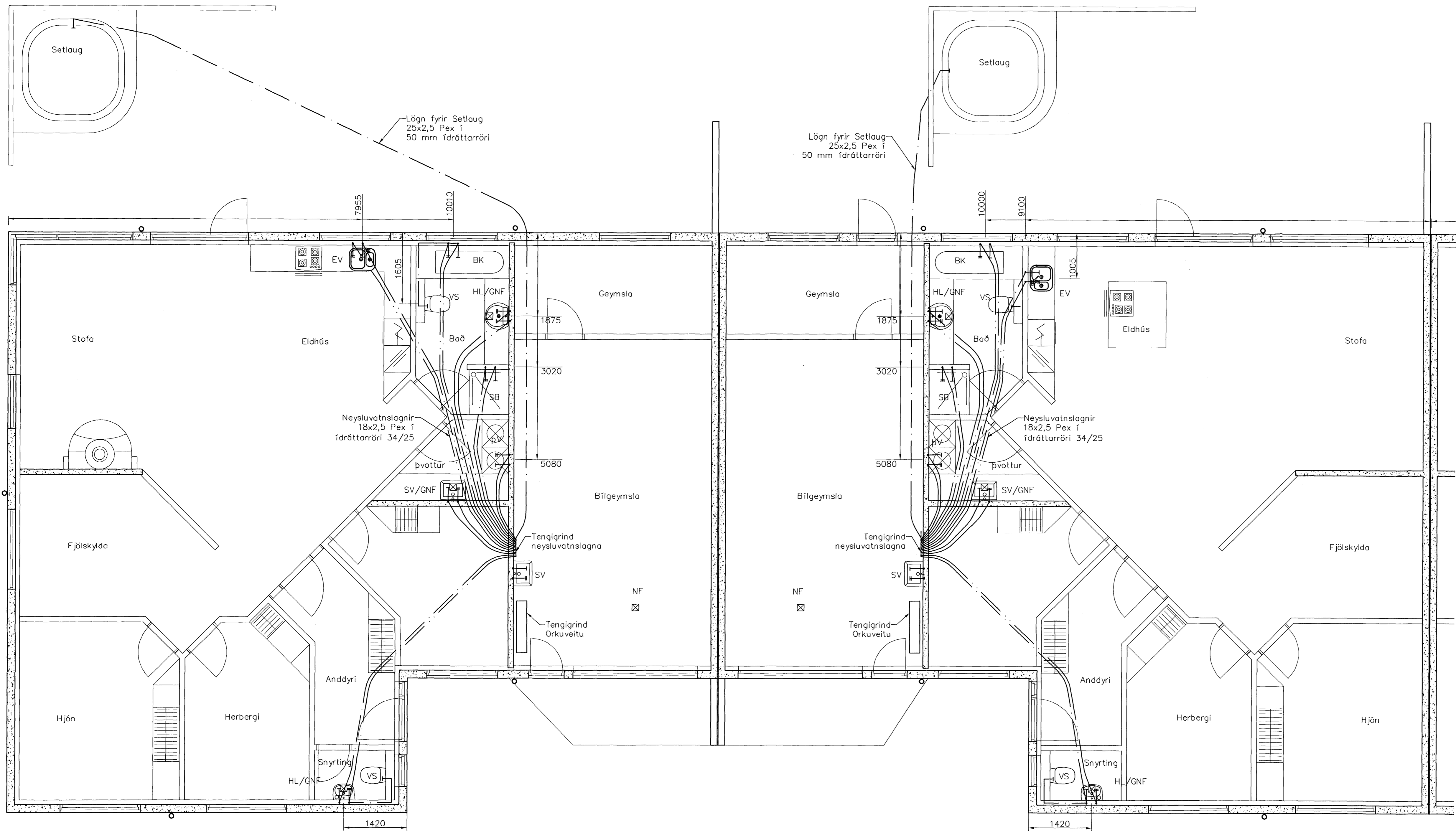
Neysluvatnslagnir 1:50
