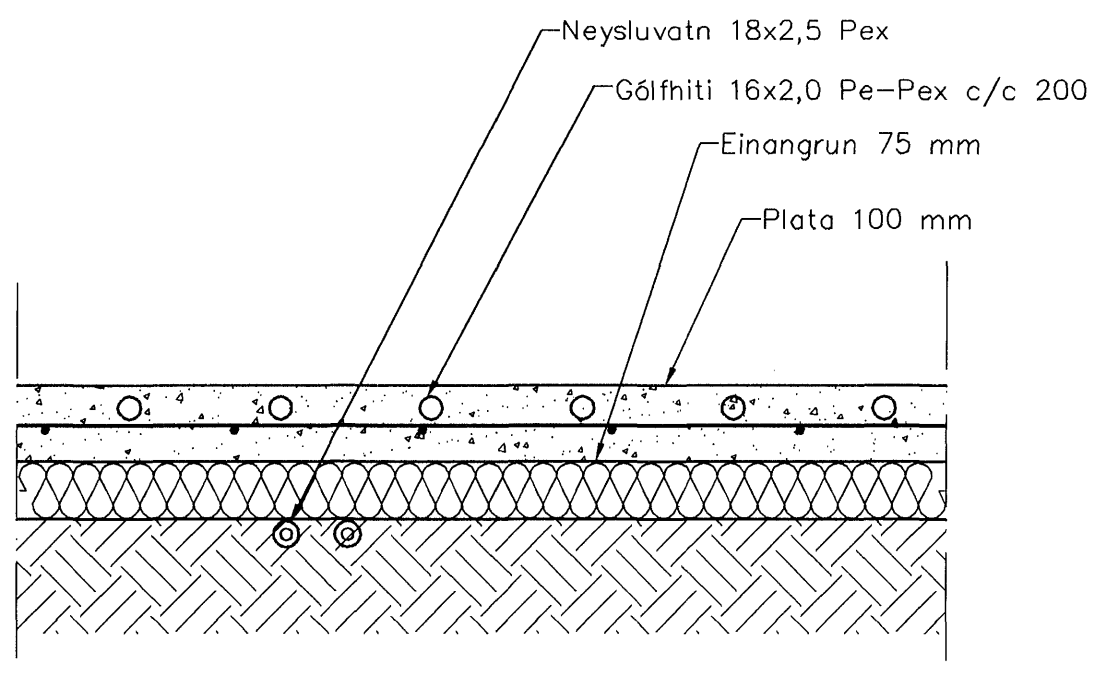
Hita- og vatnslagnir. Snið í botnplötu, fbað 1:10
