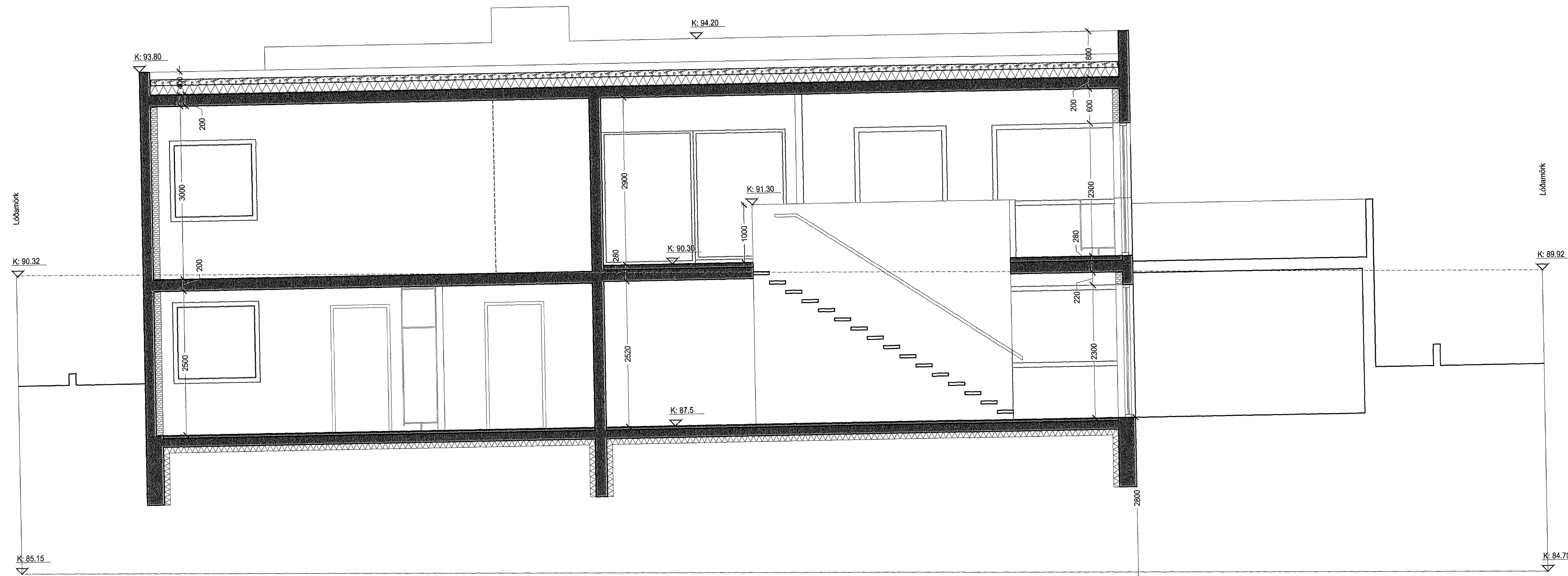
Snið B-B
