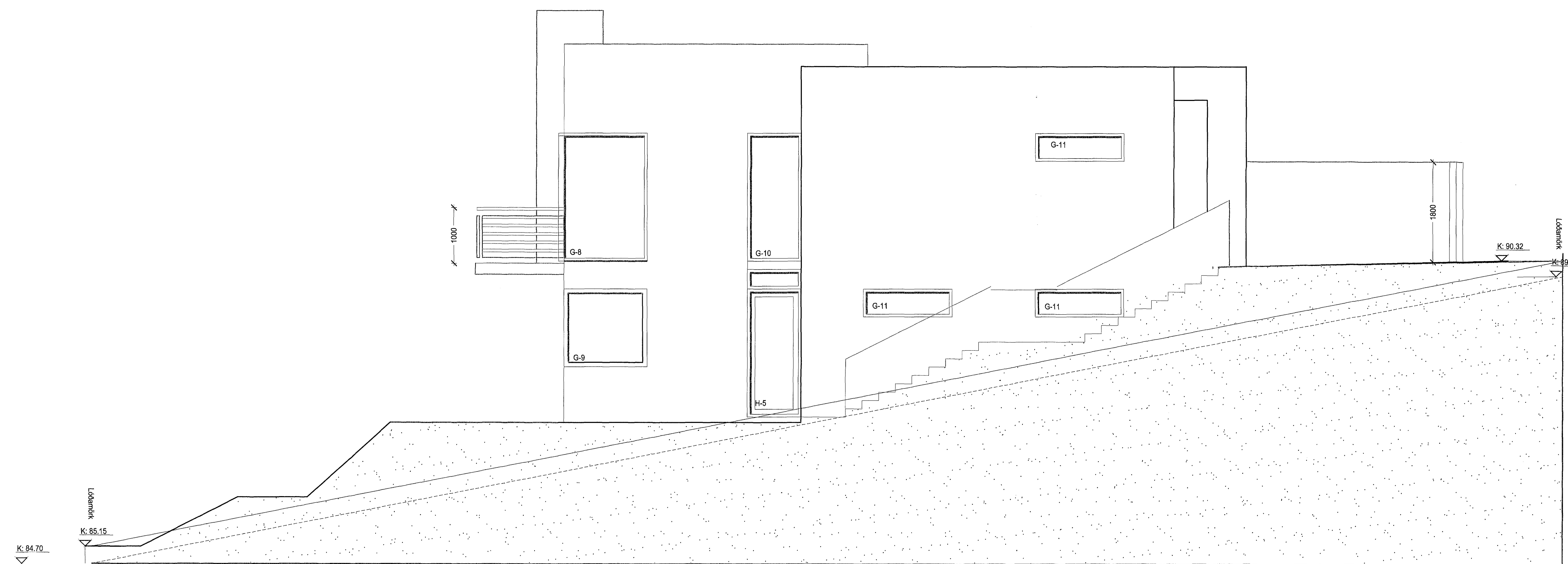
Útlit Vestur
