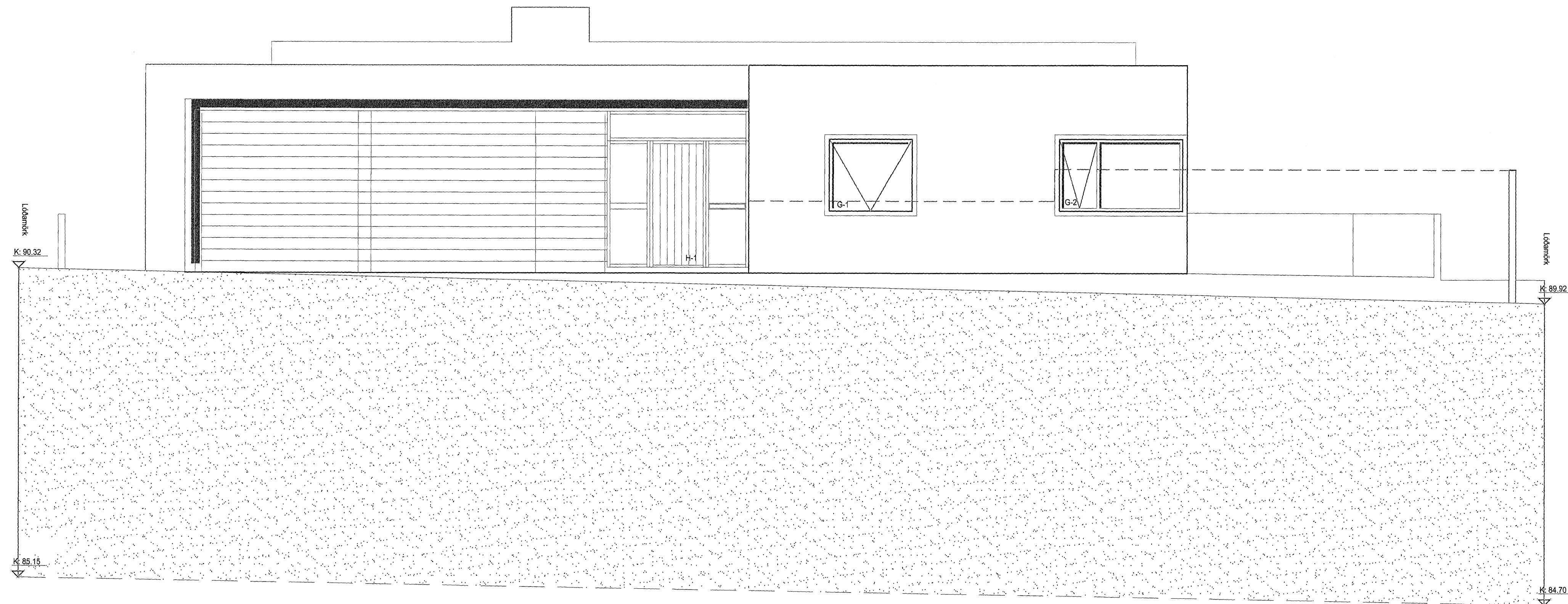
Útlit Suður
