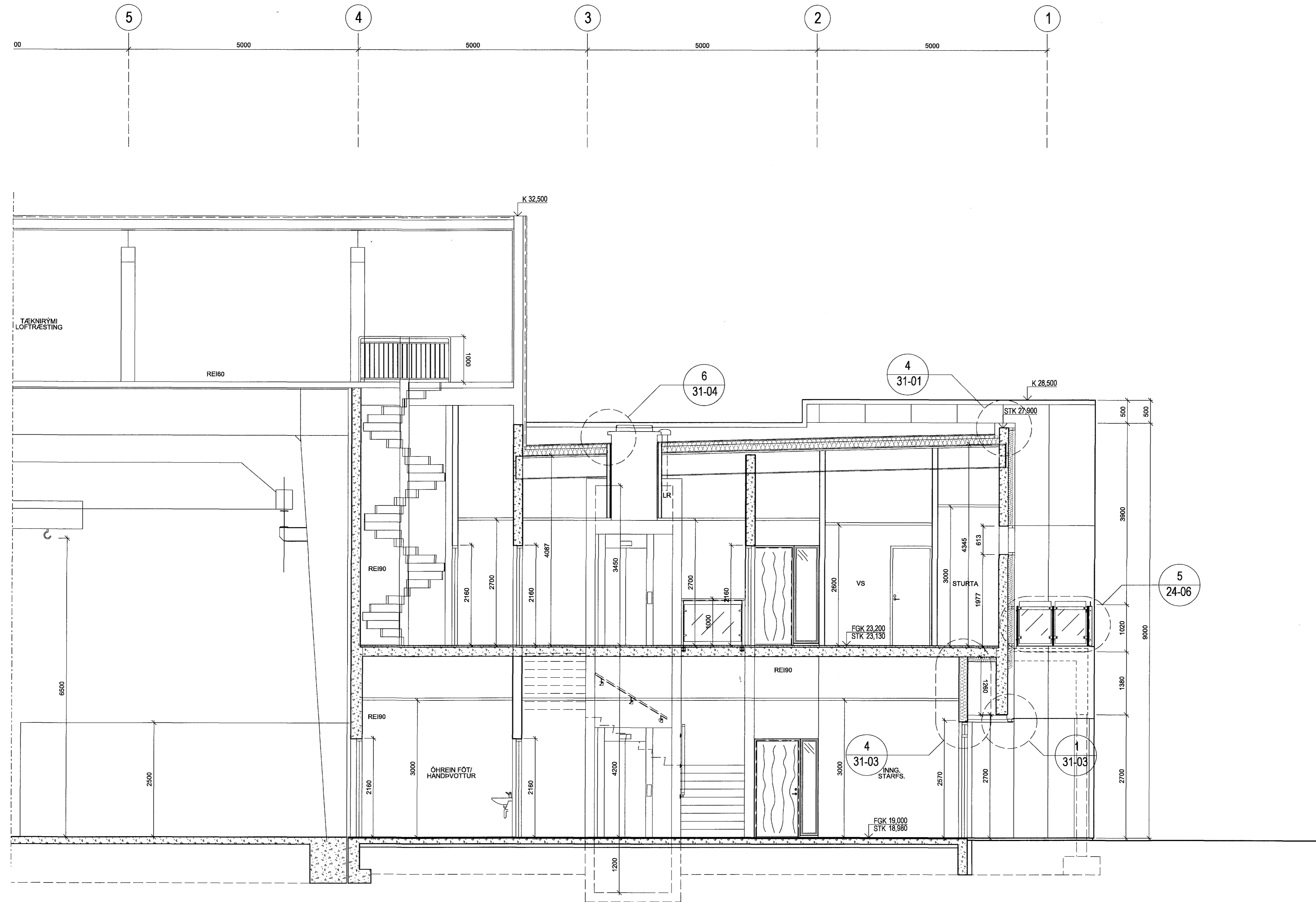
1 20-102 SNEIÐING 1:50 SKRIFSTOFUR
