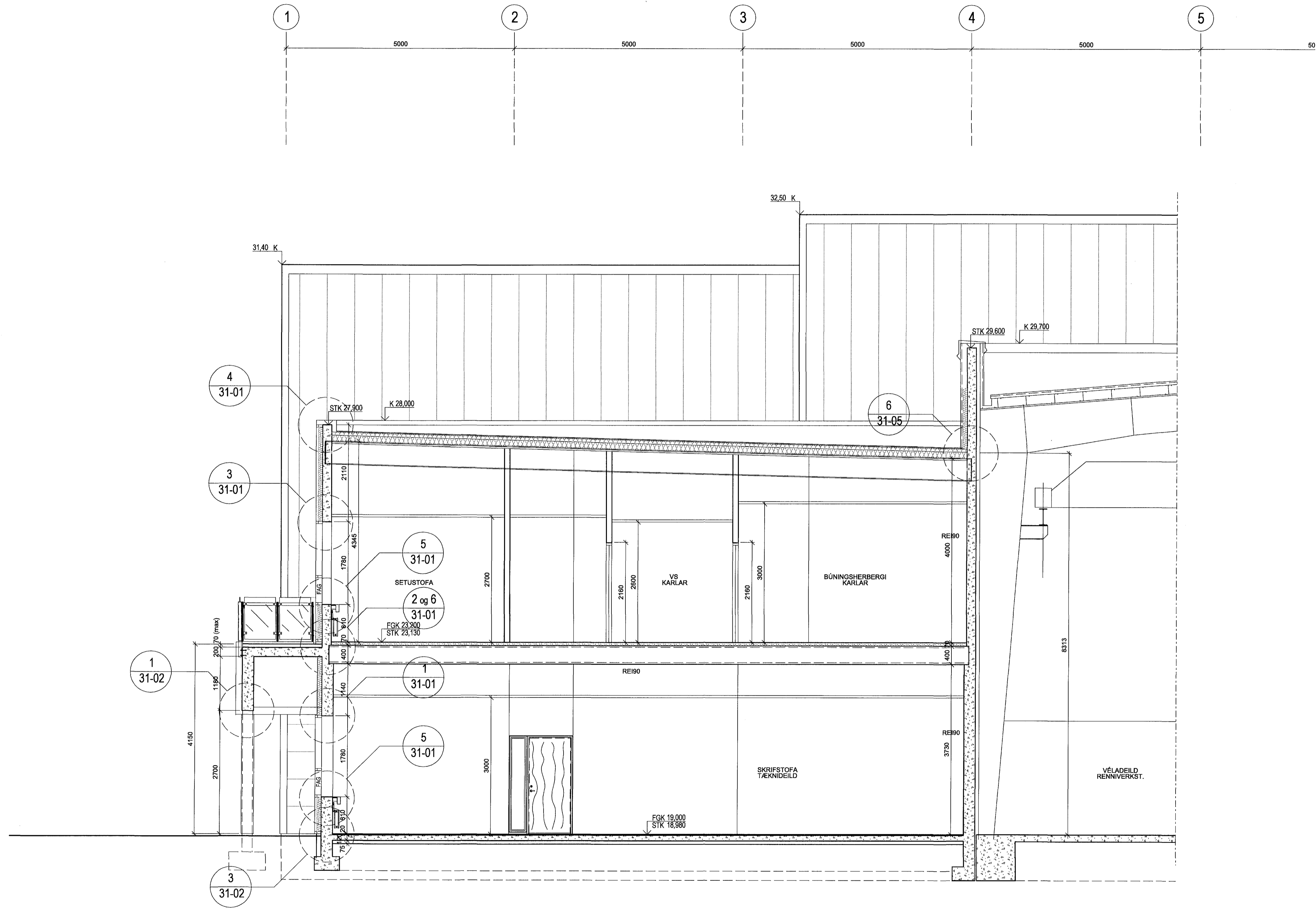
1 20-101 20-201 SNEIÐING 1:50 SKRIFSTOFUR
