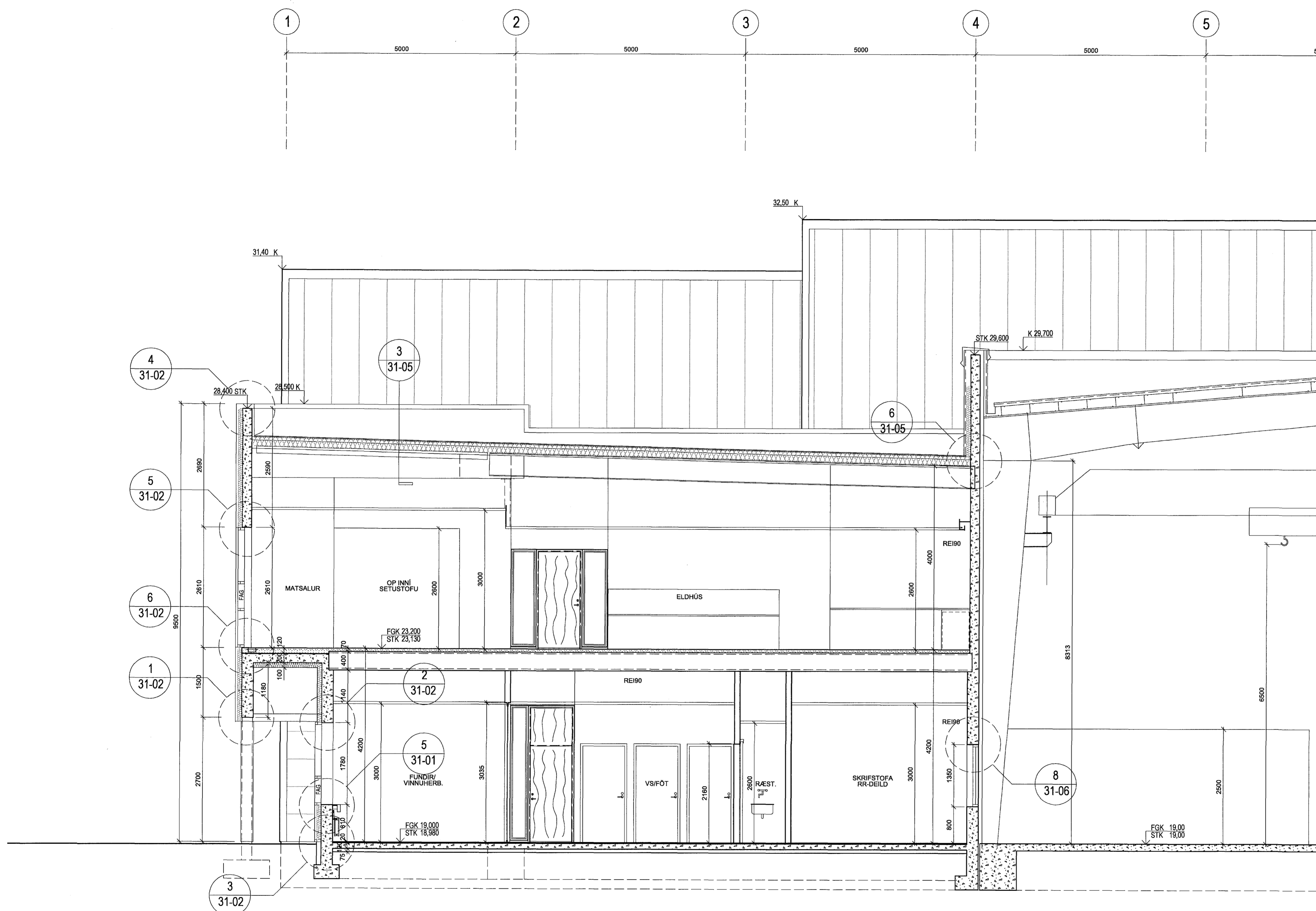
1 20-101 SNEIDING 1:50 SKRIFSTOFUR
