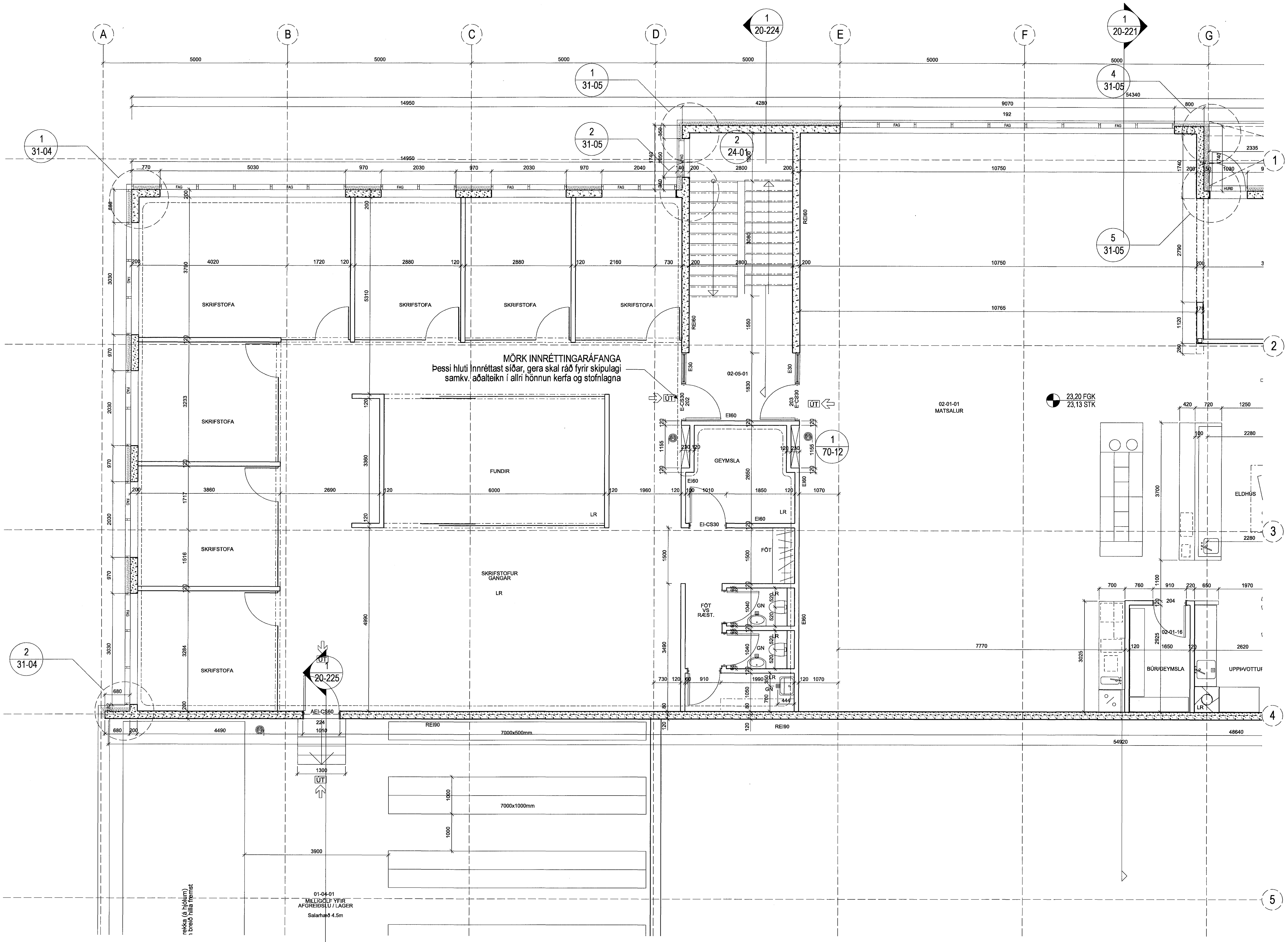
1 GRUNNMYND 2.HÆÐ (hluti 1 af 2) 1:50 Skrifstofur, matsalur, eldhús, stíghús 1
