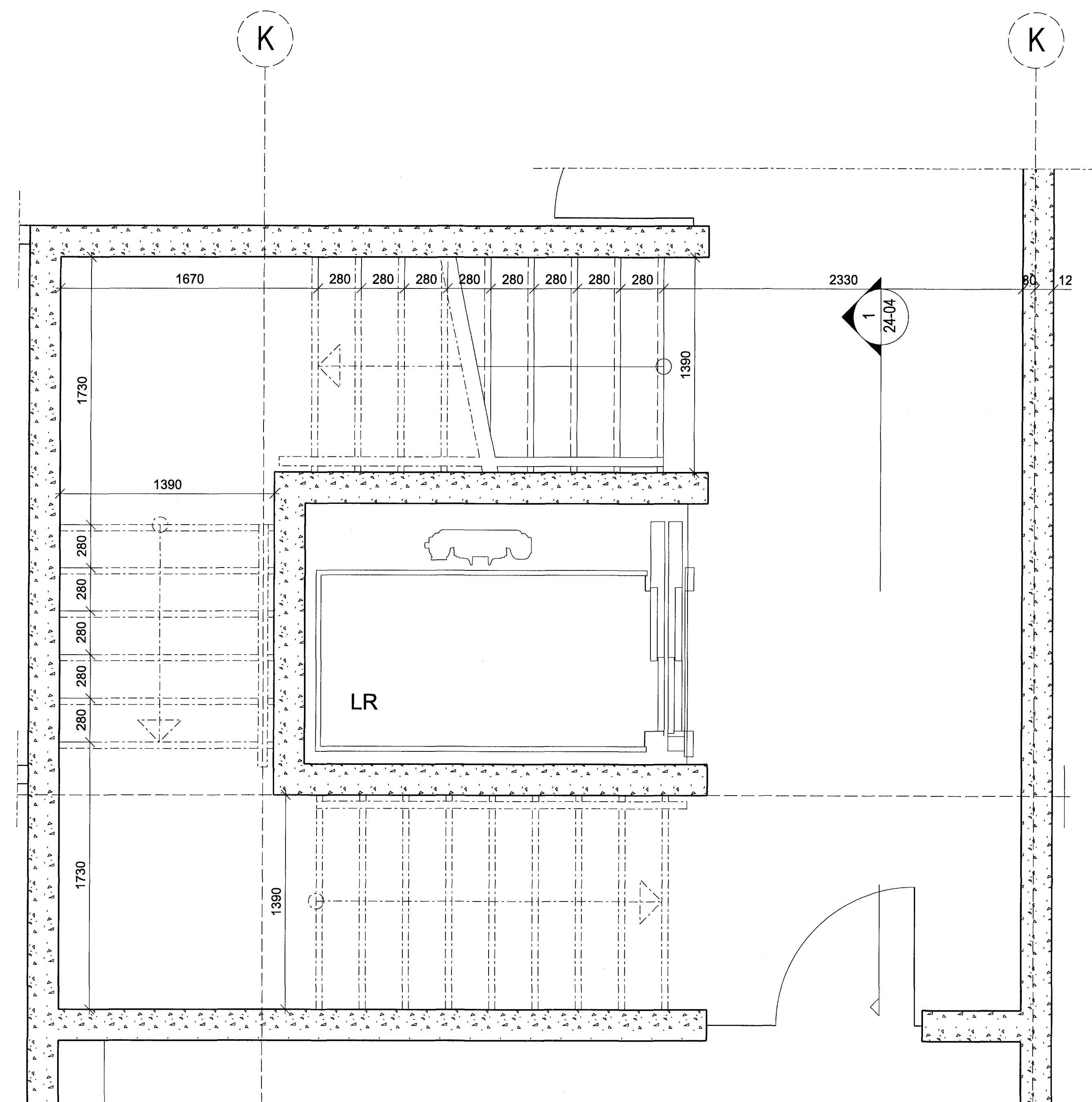
1 20-102 GRUNNMYND STIGA 1.HÆÐ 1:20 Grunnmynd stiga 1.hæð
