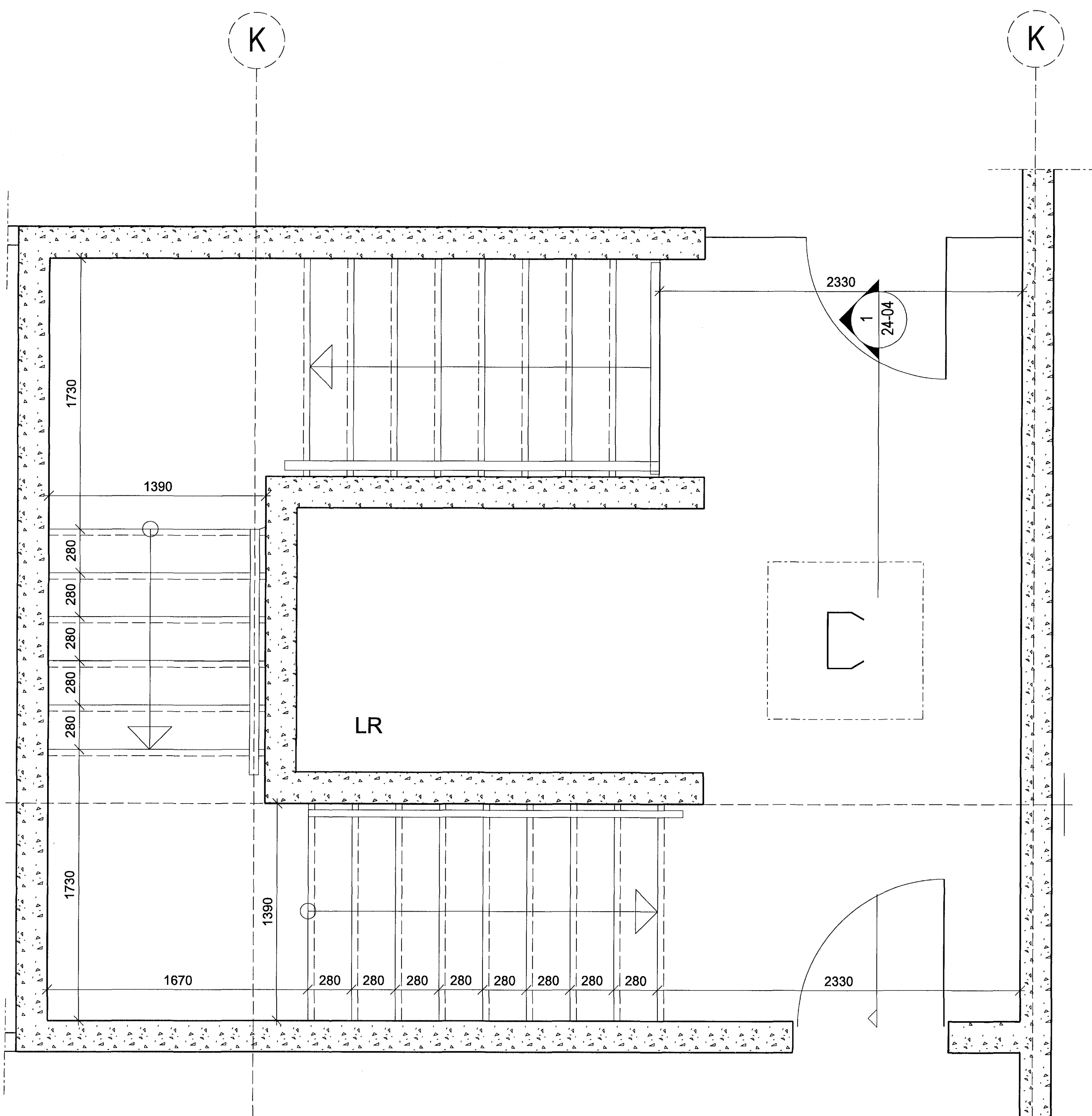
2 20-202 GRUNNMYND STIGA 2.HÆÐ 1:20 Grunnmynd stiga 2.hæð
