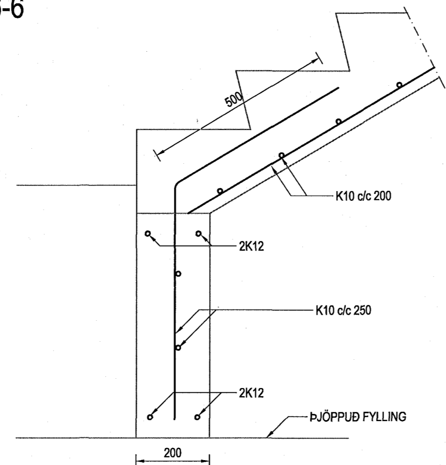
SNID 9-9 MKV. 1:10
