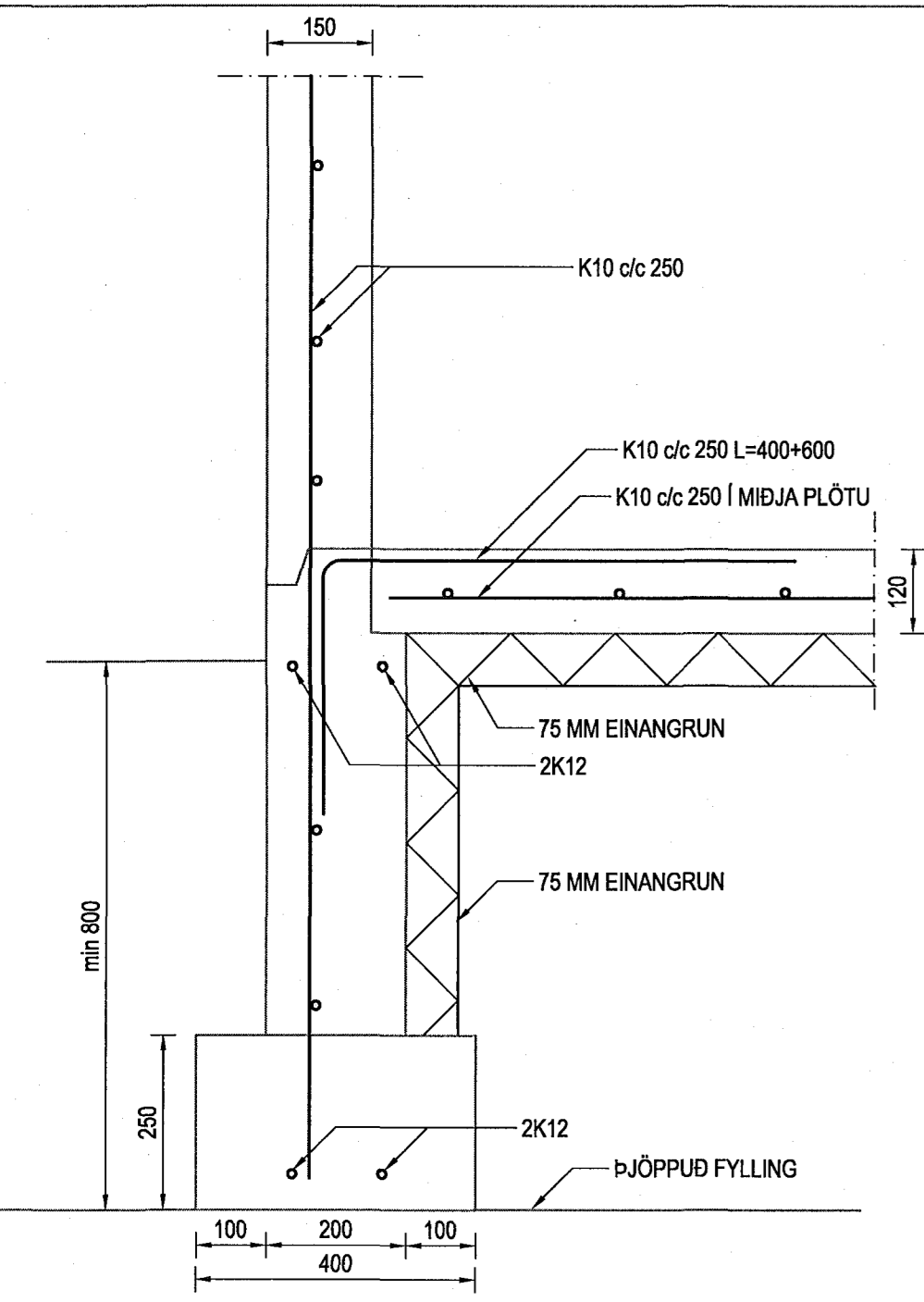
SNID 1-1 MKV. 1:10
