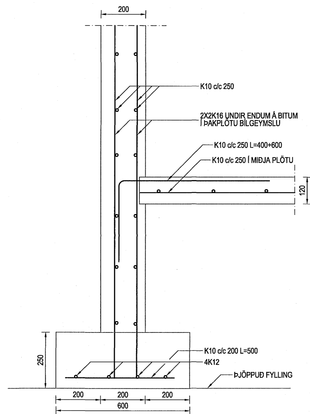
SNID 6-6 MKV. 1:10
