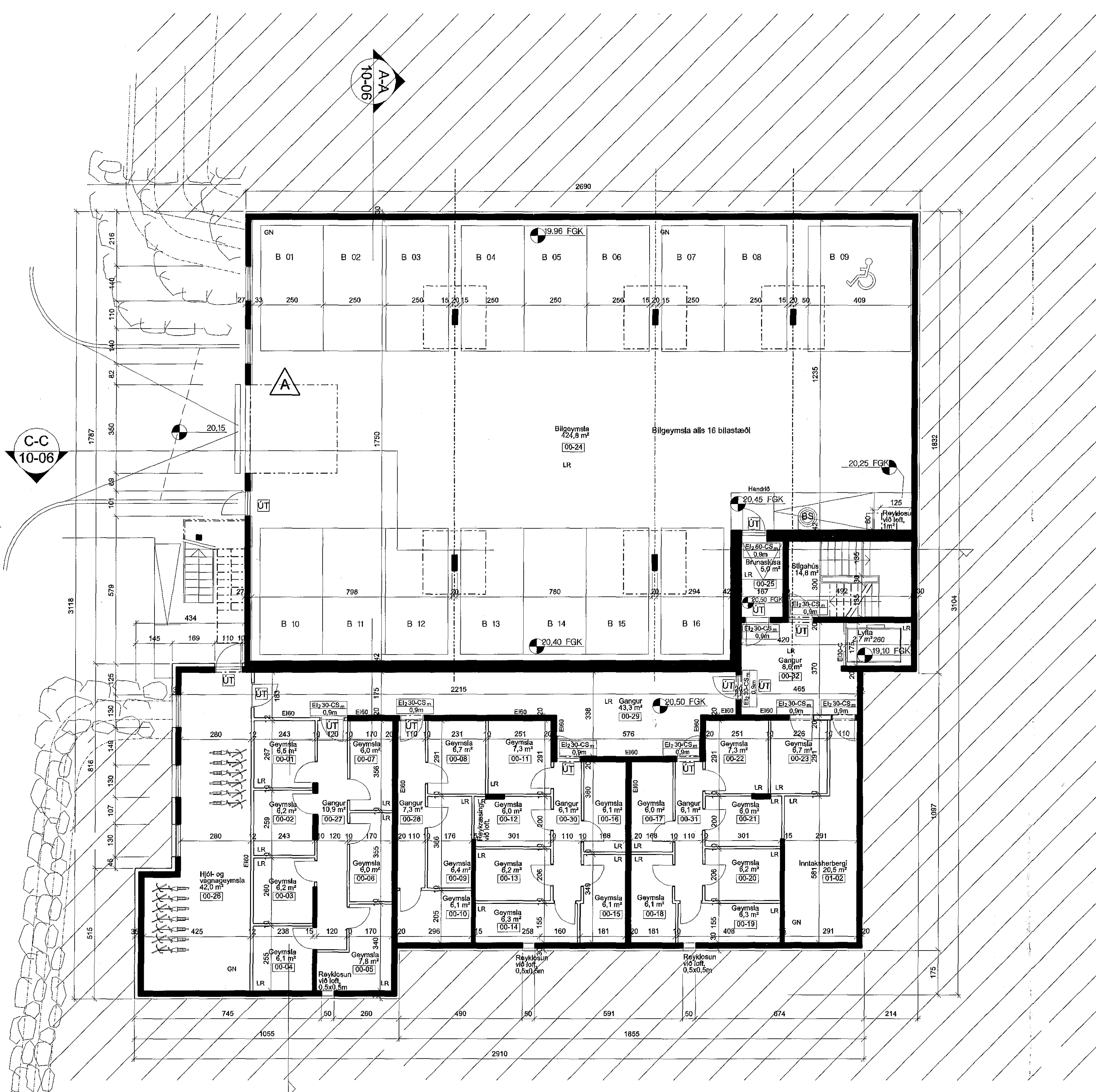
GRUNNMYND 1:100 KJALLARI
