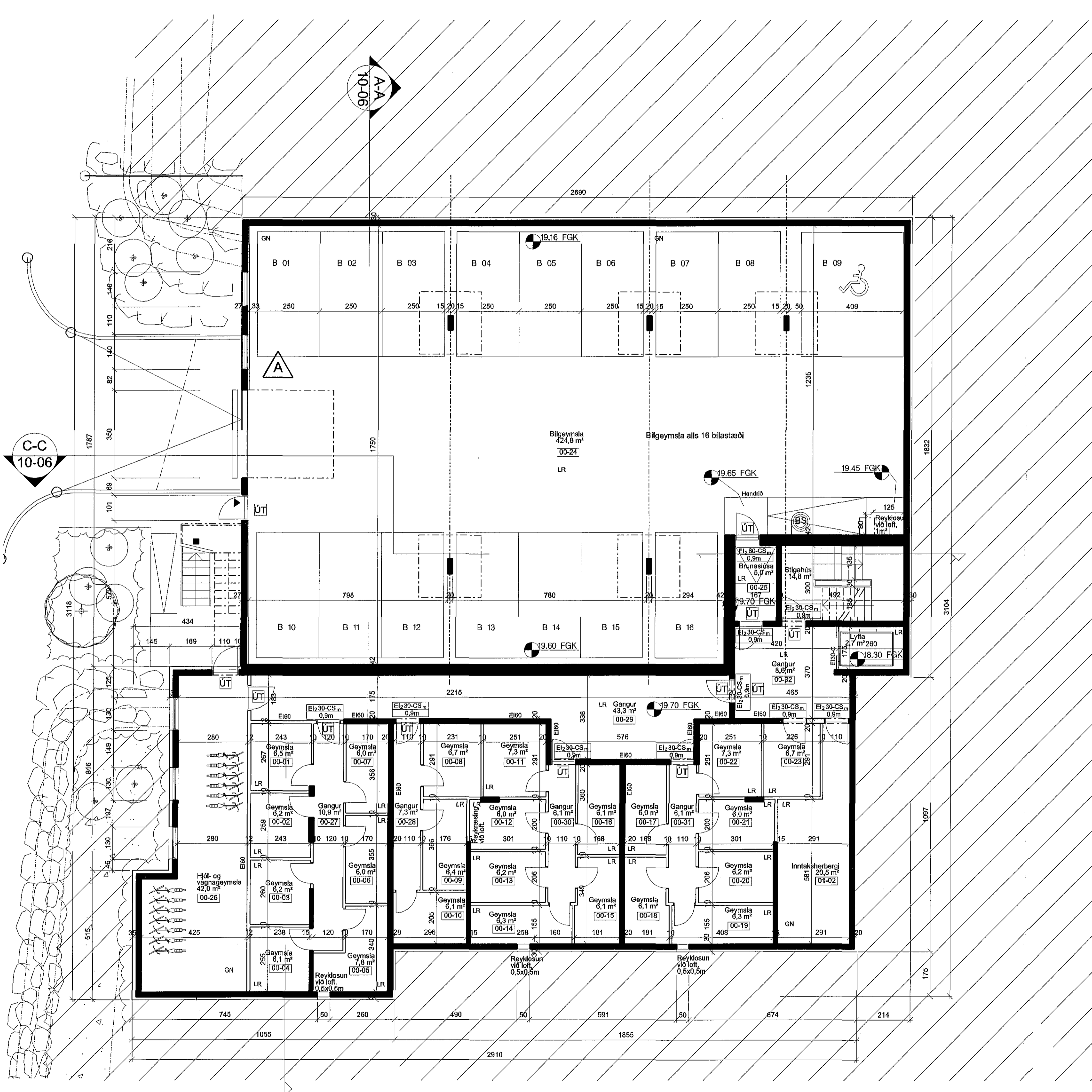
GRUNNMYND 1:100 KJALLARA
