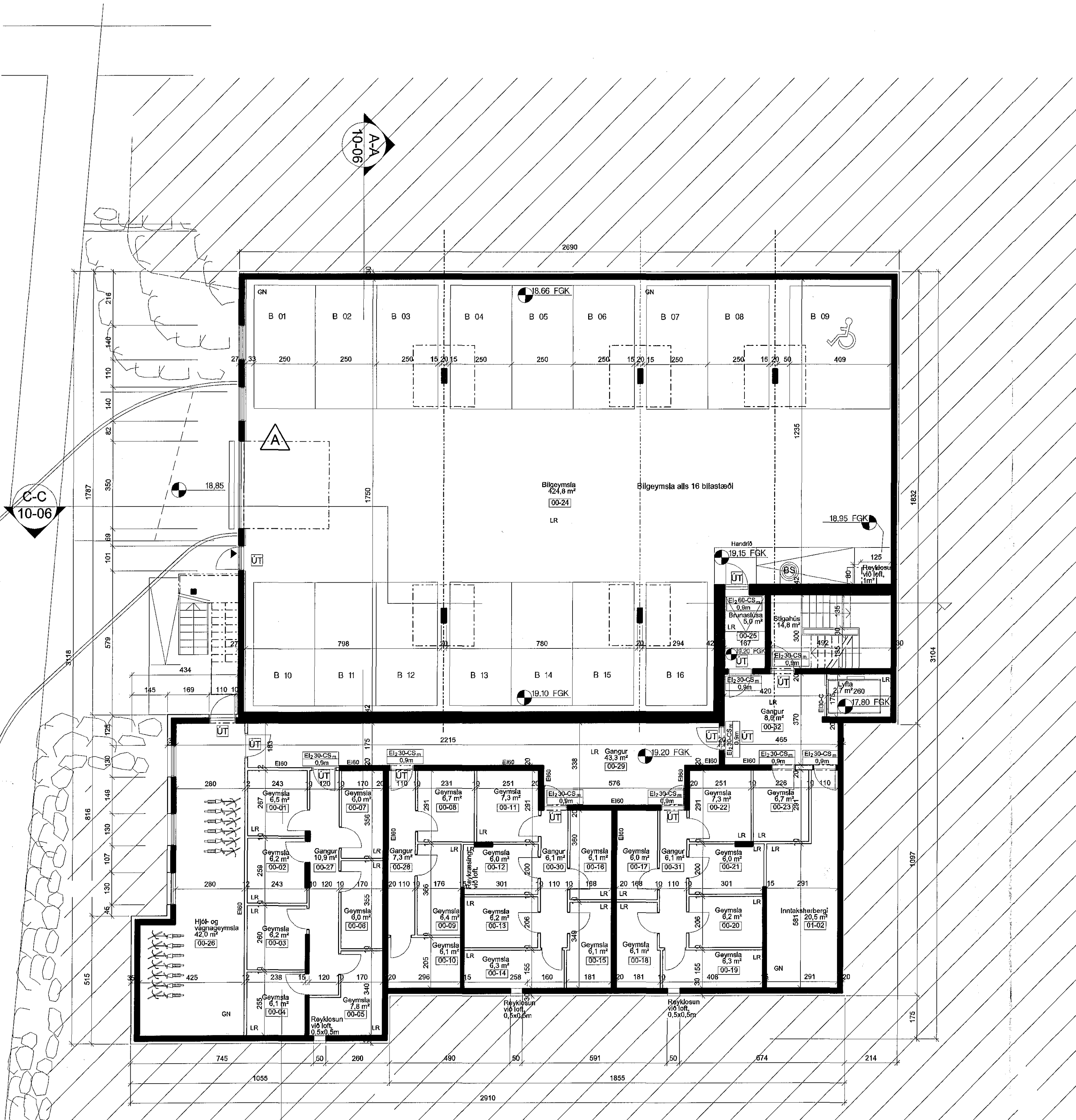
GRUNNMYND 1:100 KJALLARI
