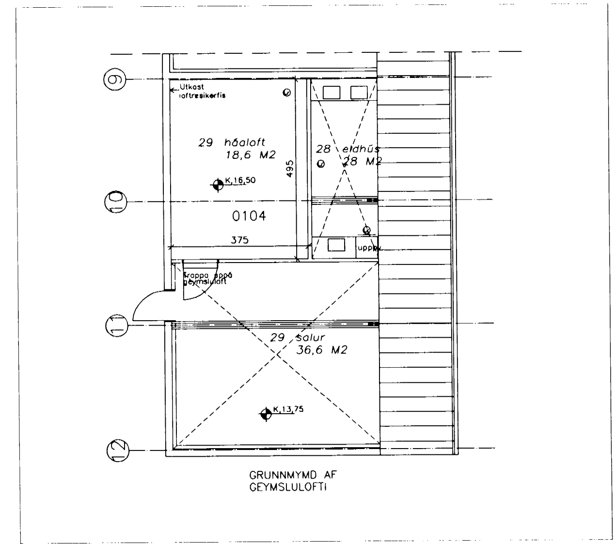
GRUNNMYND GEYMSLULOFTS
