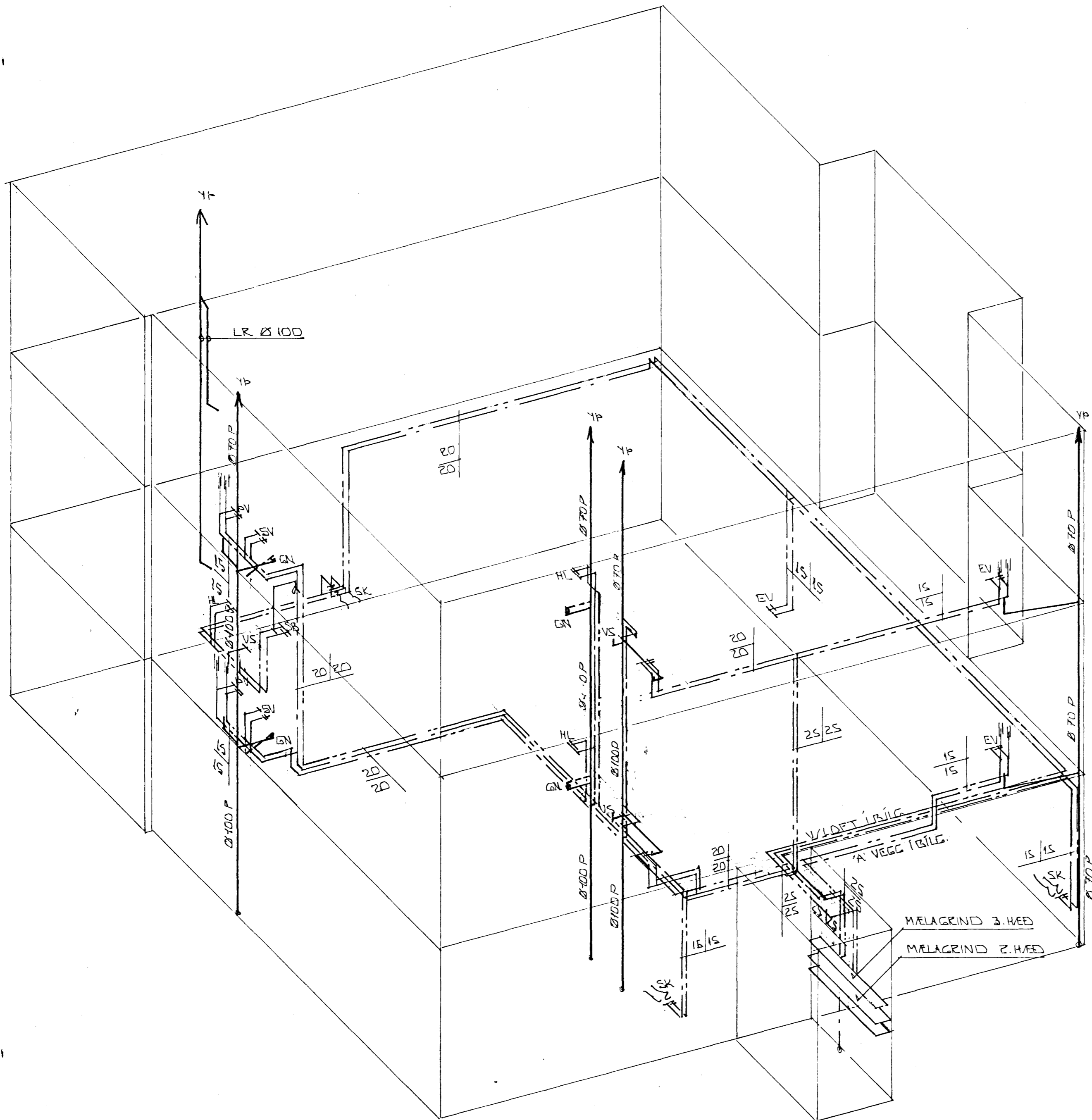
RÚMMYND VATNS- OG FRÆRENNSLISLAGNA 1:50
