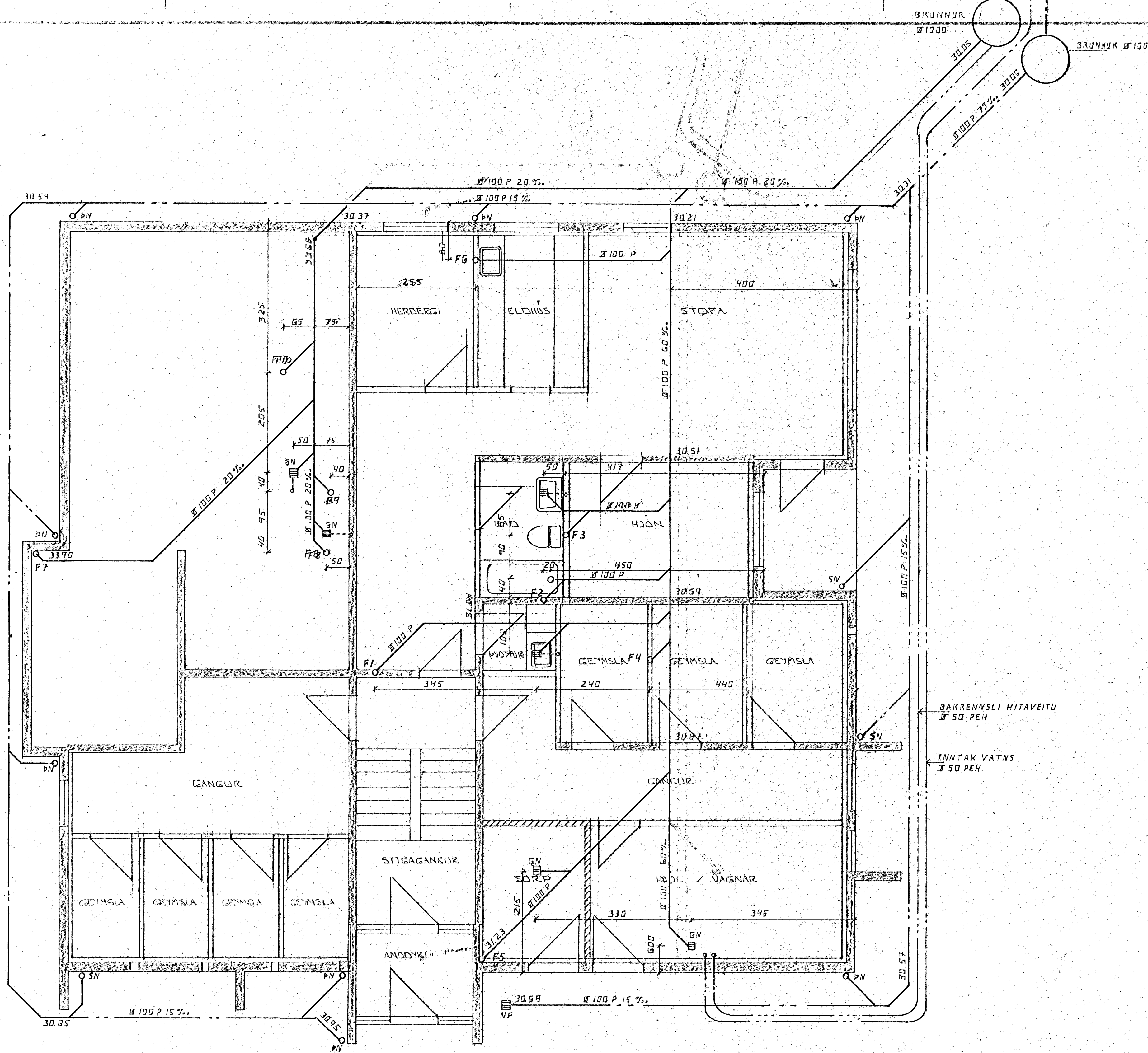
GRUNNMYND • 1:50
