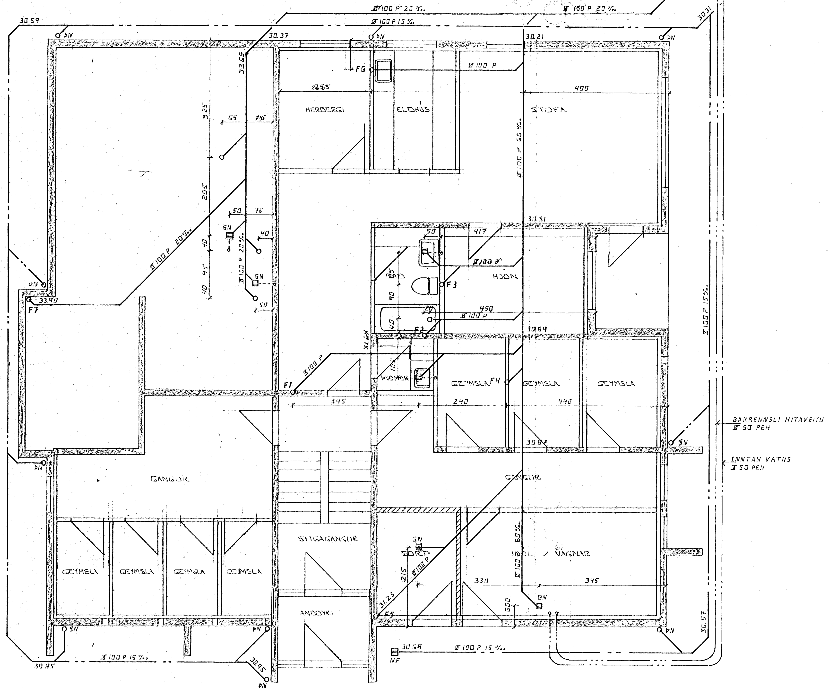
GRUNNMYND 1:50
