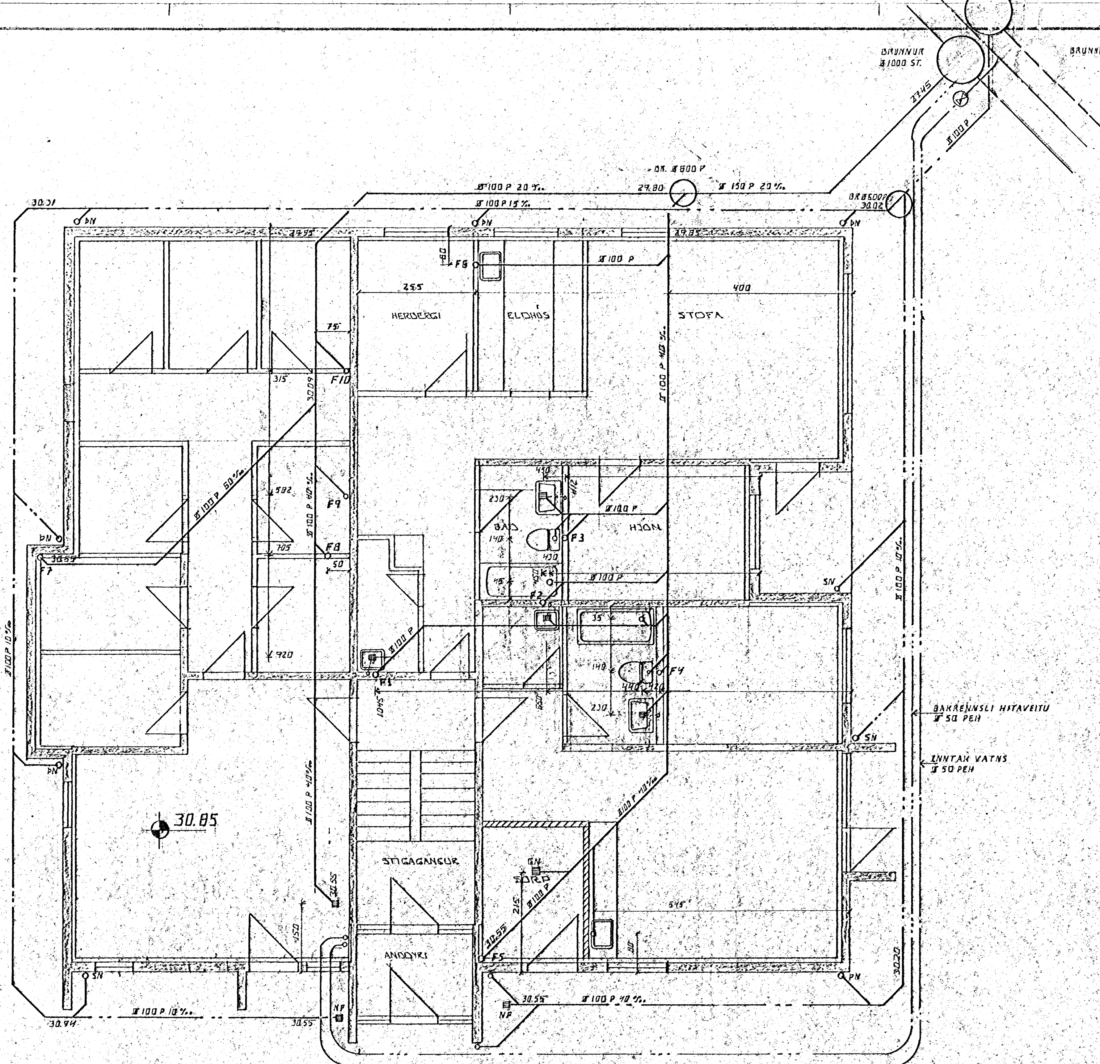
GRUNNMÝND 1:50
