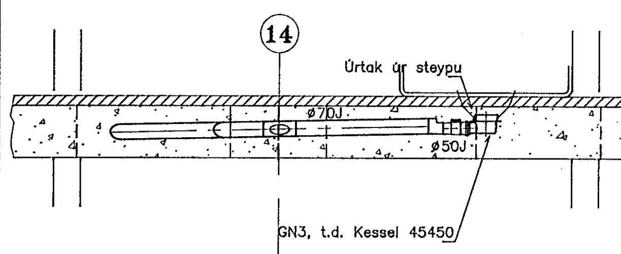
1 SNID 108/108 M. 1:20
