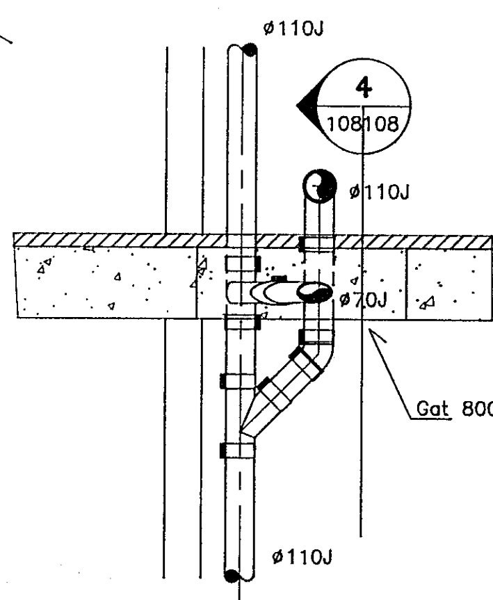
2 SNID Ekki með l uppsteypu 108/108 M. 1:20
