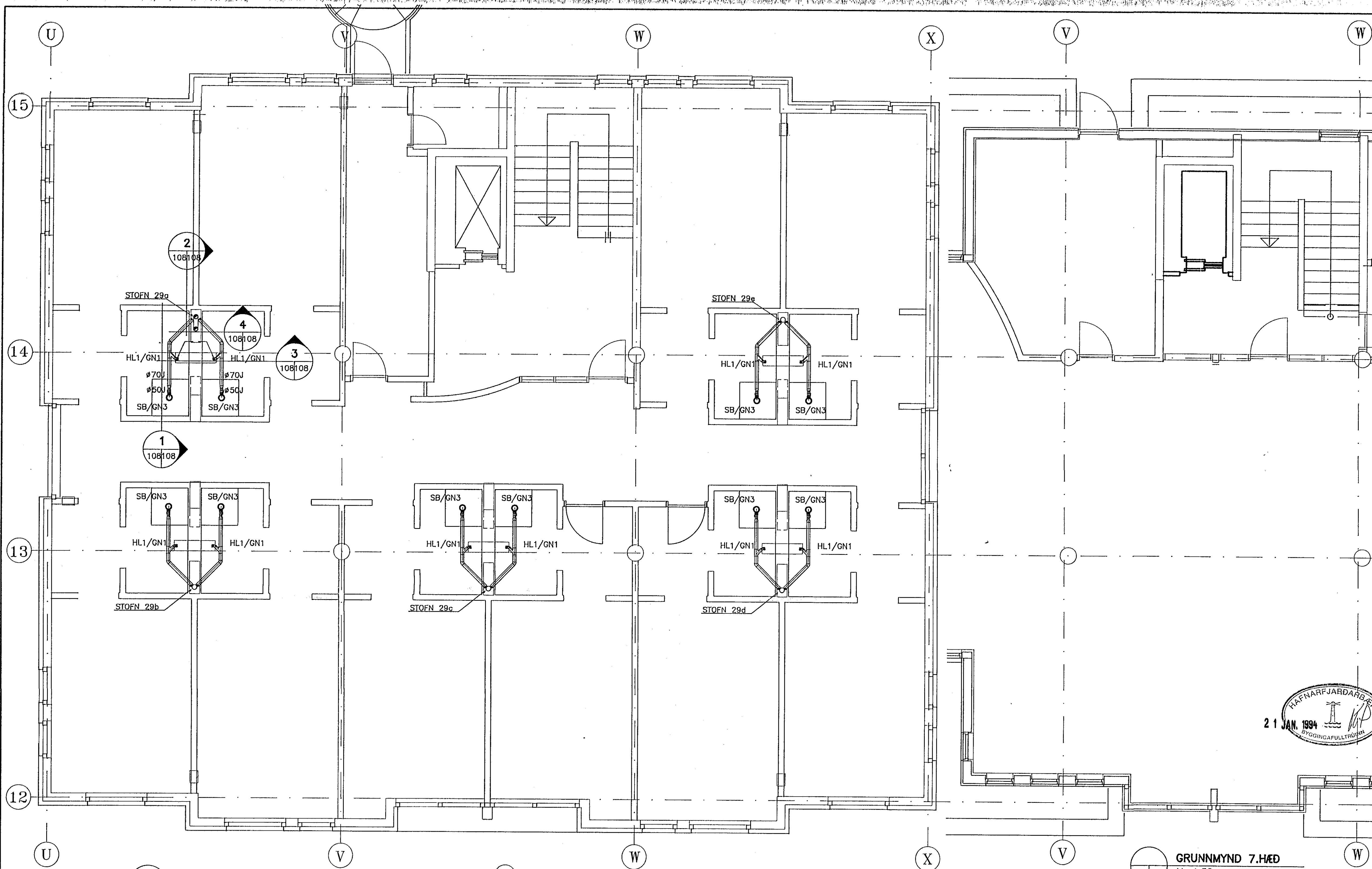
GRUNNMYND 4.-6.HÆÐ M. 1:50
