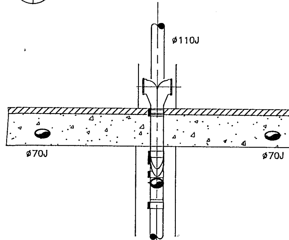
4 SNID 108/108 M. 1:20
