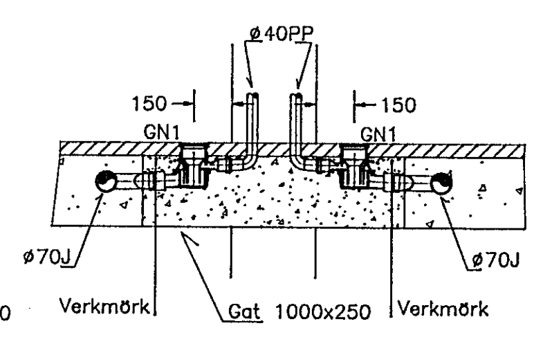
3 SNID 108/108 M. 1:20
